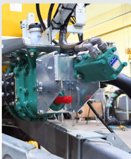
Pohon čerpadla hydromotorom
