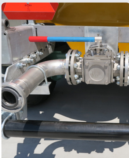
Nerezová výbava na DAM 390
